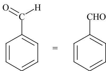
Benzaldehido Bencenocarbaldehido Formilbenceno
