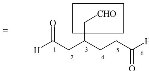
3-(Formilmetil)hexanodial
