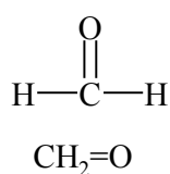
Metanal Formaldehido
