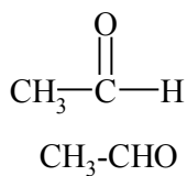
Etanal Acetaldehido
