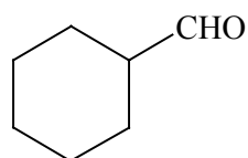
Ciclohexanocarbaldehido Formilciclohexano
