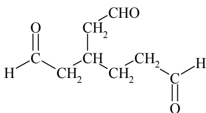
3-(Formilmetil)hexanodial
