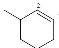
3-Metilciclohexeno
