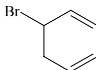
5-Bromo-1,3-ciclohexadieno
