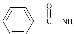
Benzamida
