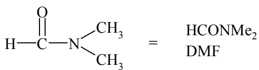
N,N -Dimetilformamida
