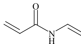
N -Vinilacrilamida
