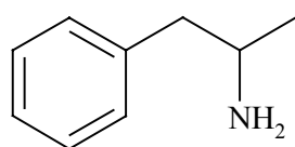
Anfetamina
