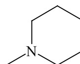
Etil metil propil amina N -Etil- N -metil-1-propanamina
