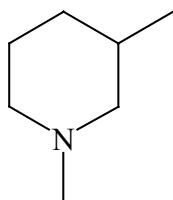
N ,3-Dimetilpiperidina
