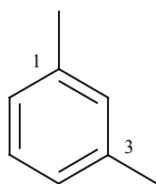
1,3-Dimetilbenceno meta -Dimetilbenceno m -Xileno
