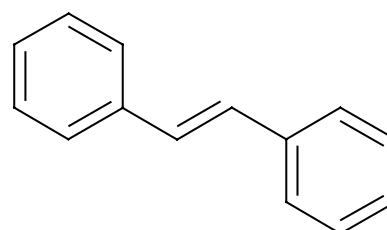
trans -Estilbeno trans -1,2-Difeniletano
