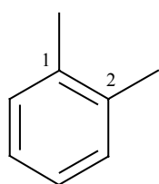
1,2-Dimetilbenceno orto -Dimetilbenceno o -Xileno
