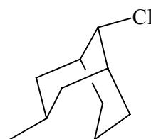
9-cloro-3-metilbiciclo[3.3.1]nonano
