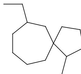
7-etil-1-metilespiro[4,6]undecano
