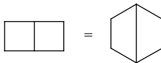
Biciclo[2.2.0]hexano
