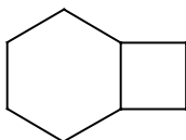
Biciclo[4.2.0]octano
