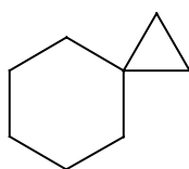
espiro[2,5]octano
