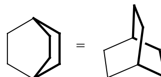
Biciclo[2.2.2]octano
