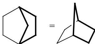
Biciclo[2.2.1]heptano
