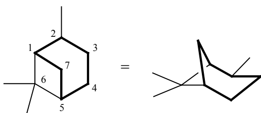
2,6,6-Trimetilbiciclo[3.1.1]heptano
