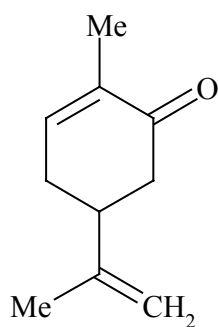
Carvona 2-Metil-5-(1-metiletenil)ciclohex-2-en-1-ona
