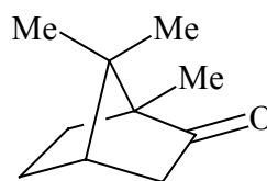
Alcanfor 1,7,7-trimetilbiciclo[2.2.1]heptan-2-ona
