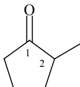
2-Metilciclopentanona
