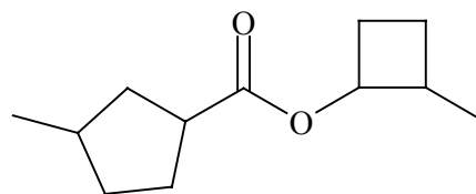
3-metilciclopentanocarboxilato de 2-metilciclobutilo
