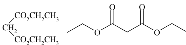
Malonato de dietilo Propanodioico dietil ester
