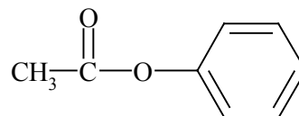
Acetato de fenilo Etanoato de fenilo
