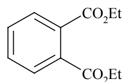
Ftalato de dietilo
