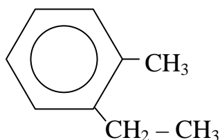
o-etilmetilbenceno/1,2-etilmetilbenceno o-ethylmethylbenzene/1,2-ethylmethylbenzene
