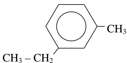
m-etilmetilbenceno/1,3-etilmetilbenceno m-ethylmethylbenzene/1,3-ethylmethylbenzene
