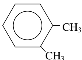
o-dimetilbenceno/1,2-dimetilbenceno o-dimethylbenzene/1,2-dimethylbenzene
