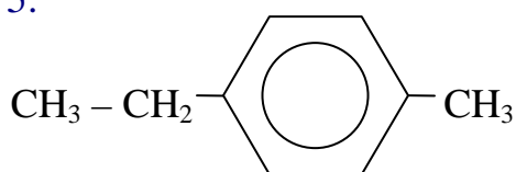
p-etilmetilbenceno/1,4-etilmetilbenceno p-ethylmethylbenzene/1,4-ethylmethylbenzene
