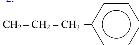
Propilbenceno Propylbenzene
