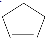
Ciclopenteno Cyclopentene
