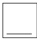
Ciclobutino Cyclobutene
