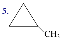
metilciclopropano
